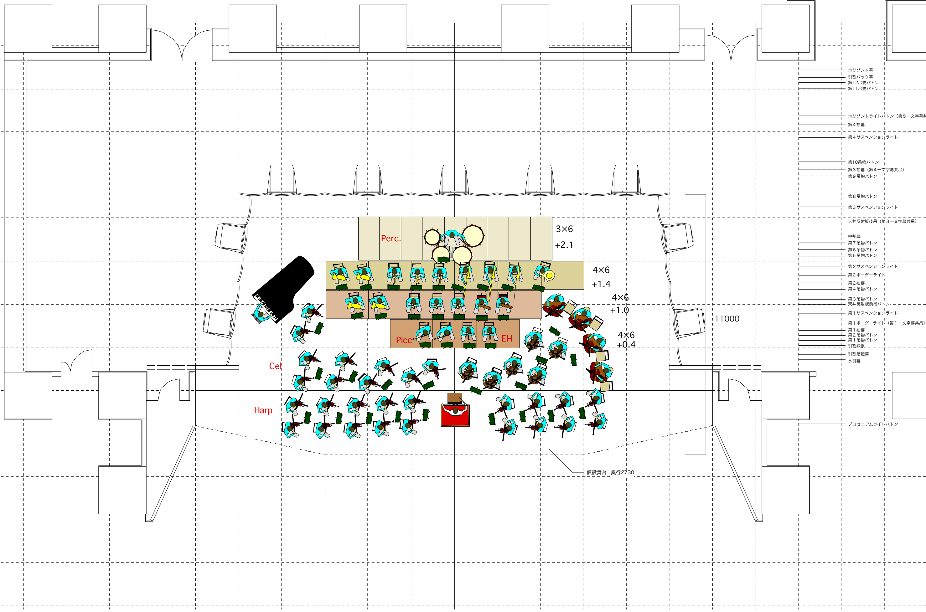
南陽市文化会館 舞台平面図 (A3 : 1 / 100)
